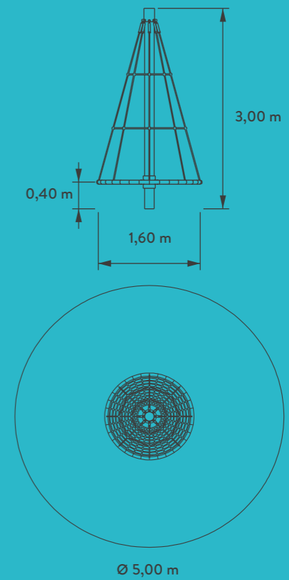
TYP N ART. 0106 – MIT VOLLFLÄCHIGEM NETZBODEN | WITH FULL NET BASE
