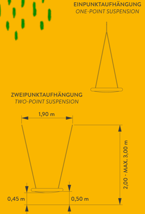
AUFHÄNGEVARIANTEN NESTSCHAUKELN SUSPENSION OPTIONS FOR NEST SWINGS
