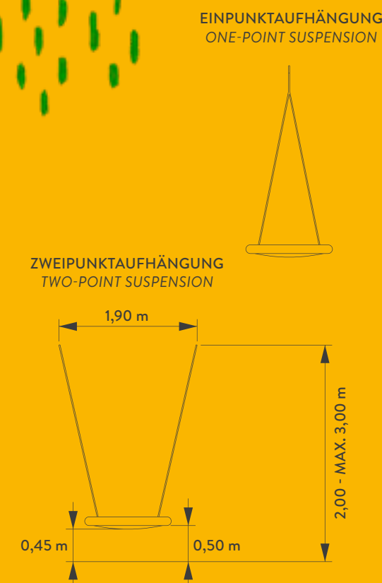
AUFHÄNGEVARIANTEN NESTSCHAUKELN SUSPENSION OPTIONS FOR NEST SWINGS
